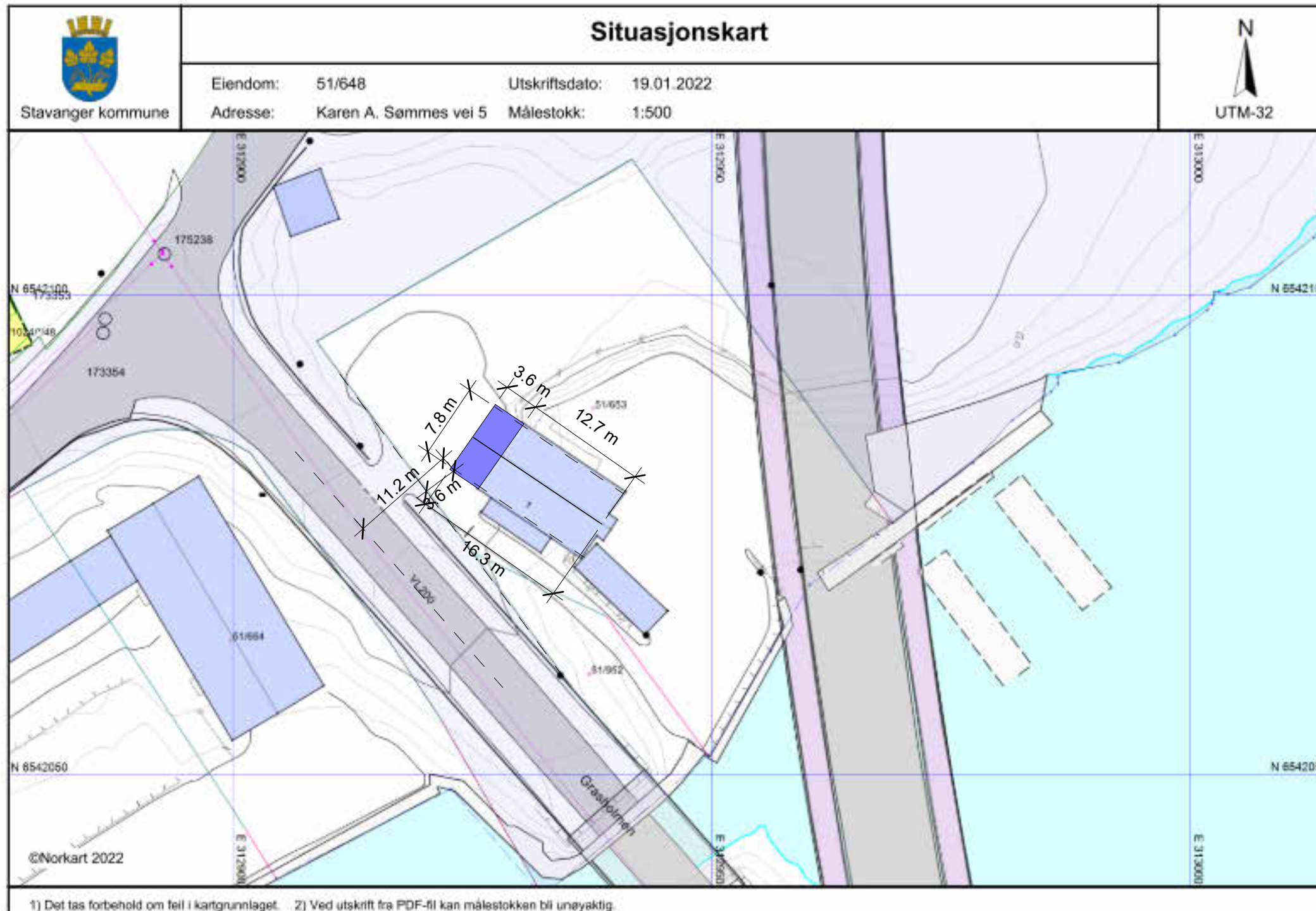
Situasjonsplan 1 : 500
